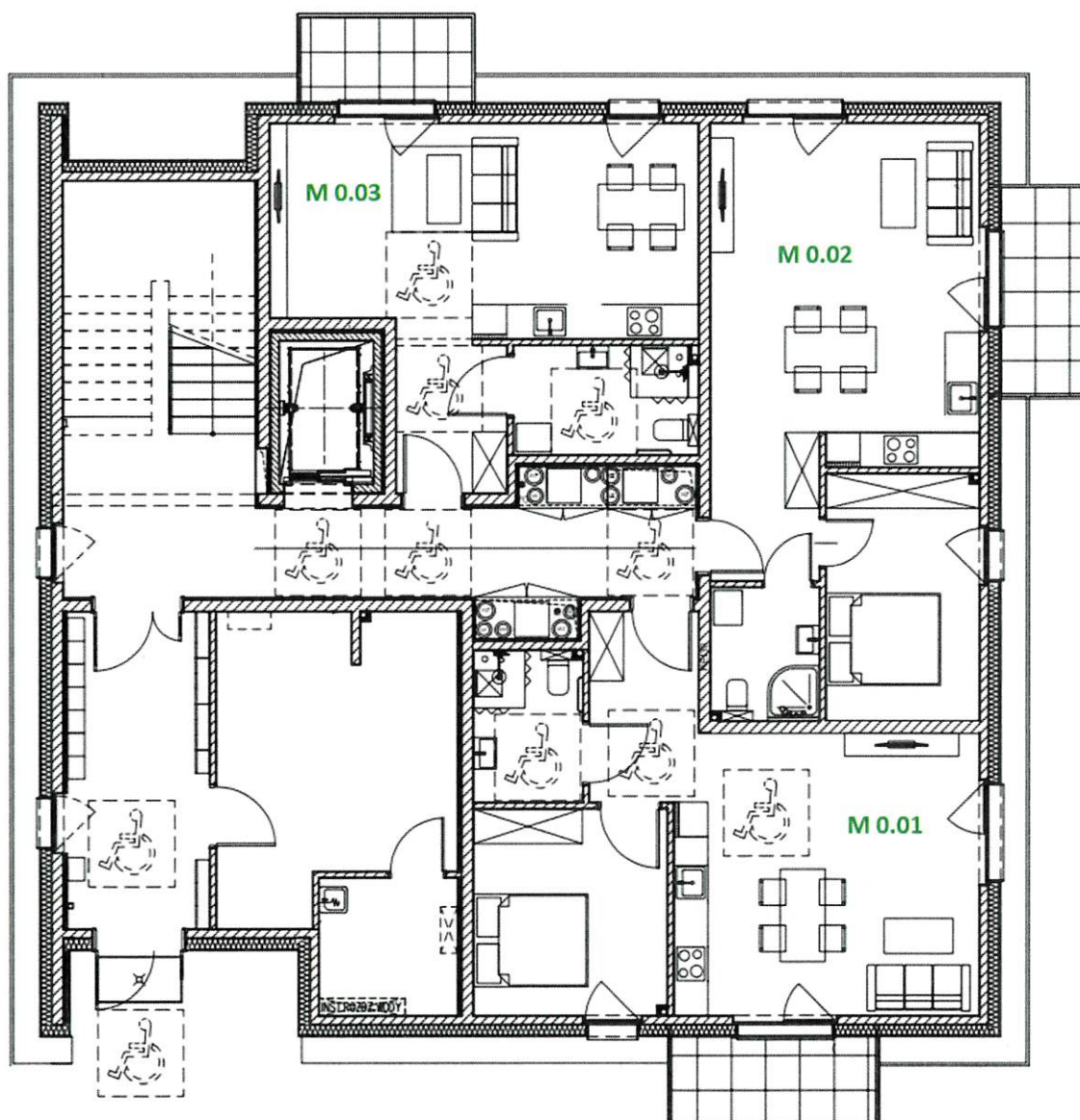
RZUT PARTERU
