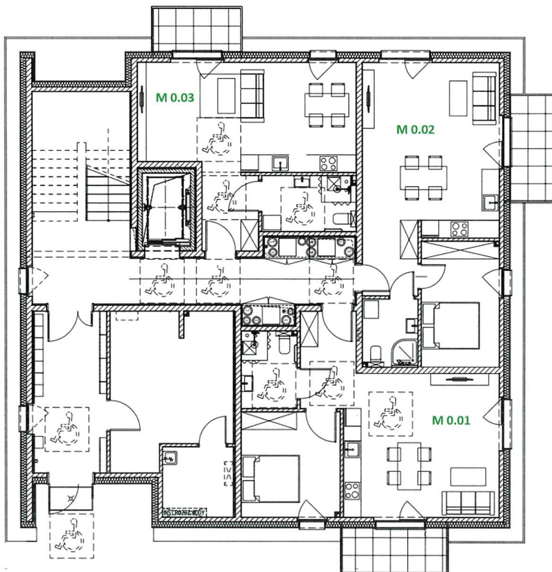
RZUT PARTERU
